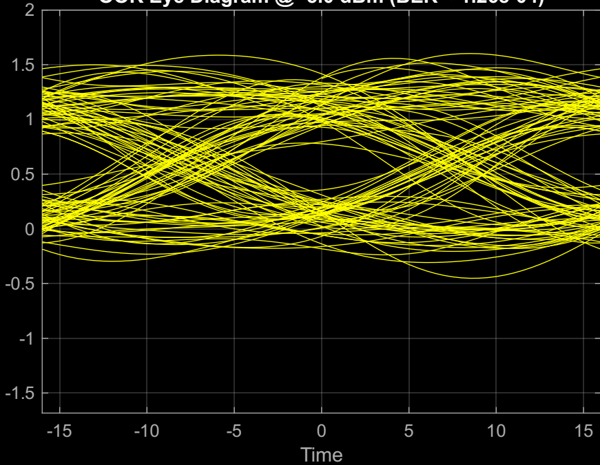
OOK Eye Diagram @ -5.0 dBm (BER \approx 1.26\text{e-}04 )
